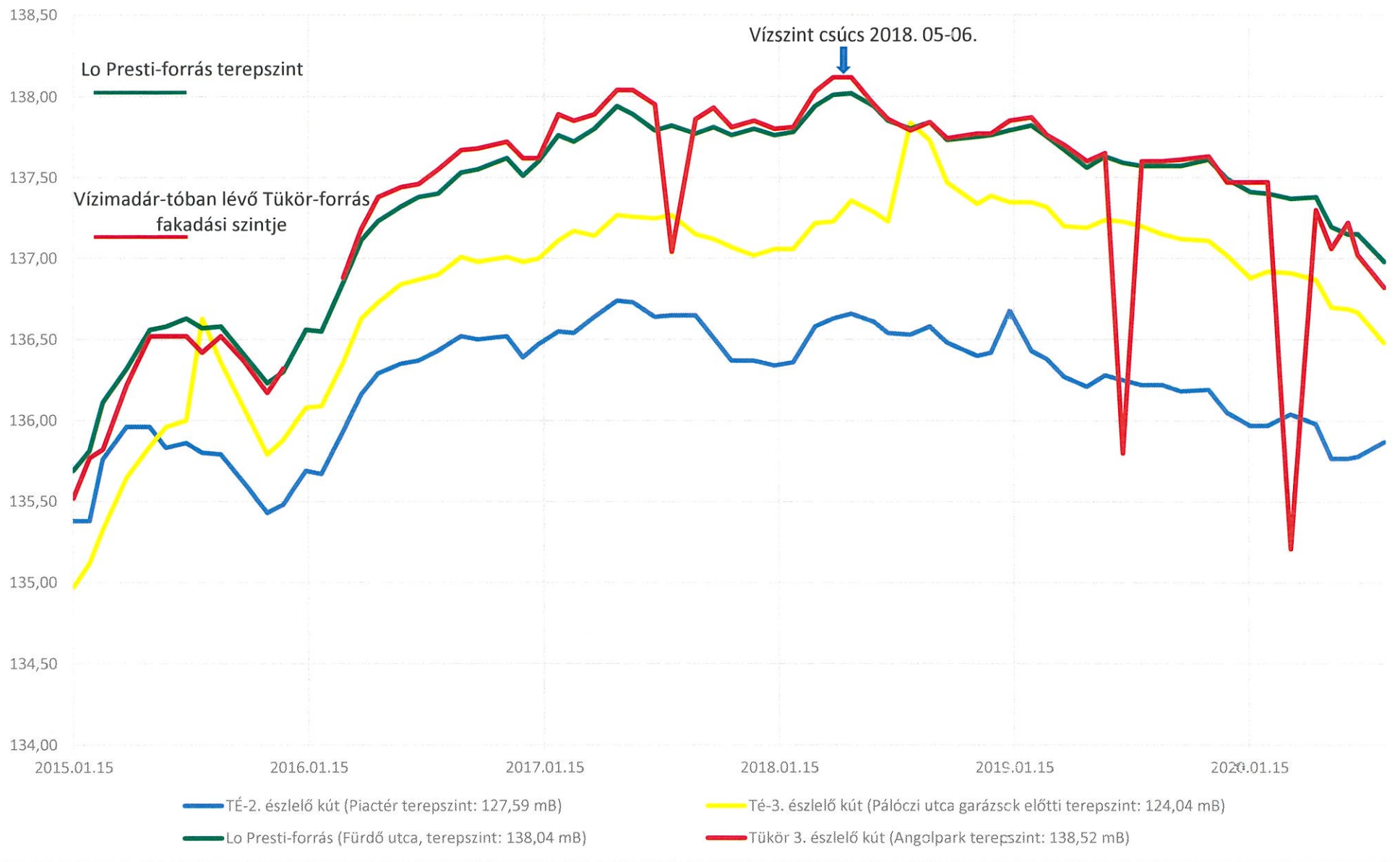
Tata karsztvízszint alakulása (2015. 01. 15. - 2020. 08. 12.)
