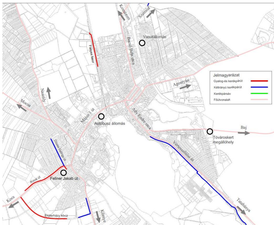
65. ábra: Meglévő kiépített kerékpáros vonali létesítmények Tatán (2014)
